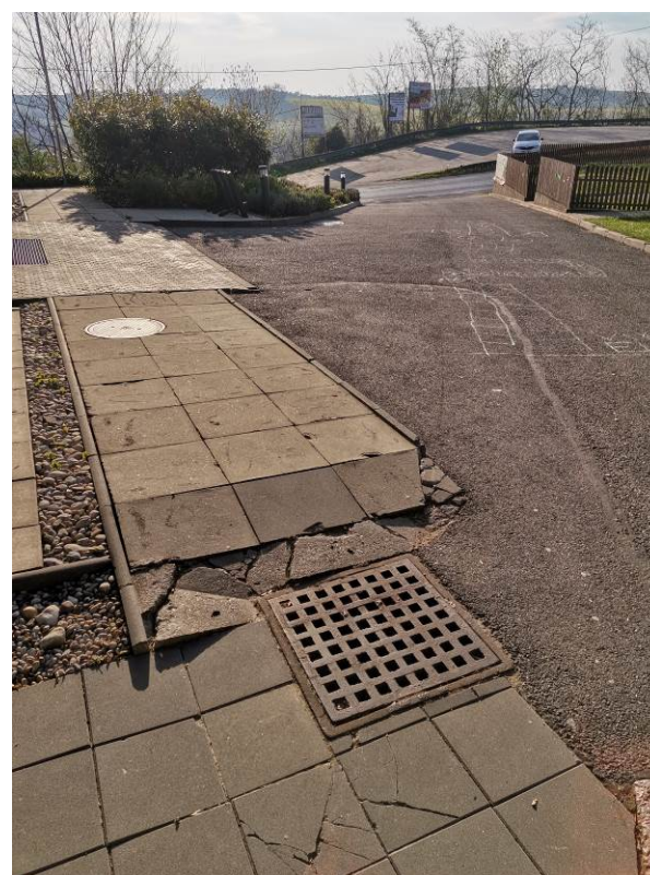
nápojení vpustí do stoky C.1
