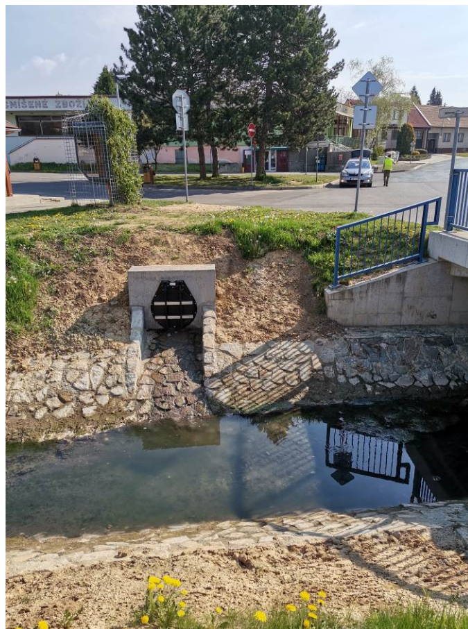
Vyústění stoky A
